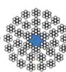
37 x 7+FC
