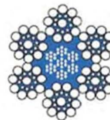
6 x 19S+IWRC
