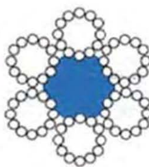
6 x 12+7FC
