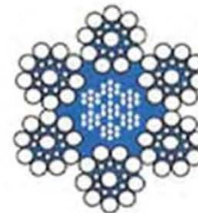
6 x 19S+IWRC
