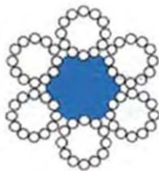
6 x 12+7FC
