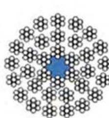
37 x 7+FC
