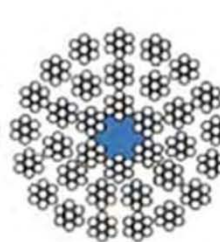
37 x 7+FC
