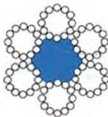
6 x 12+7FC
